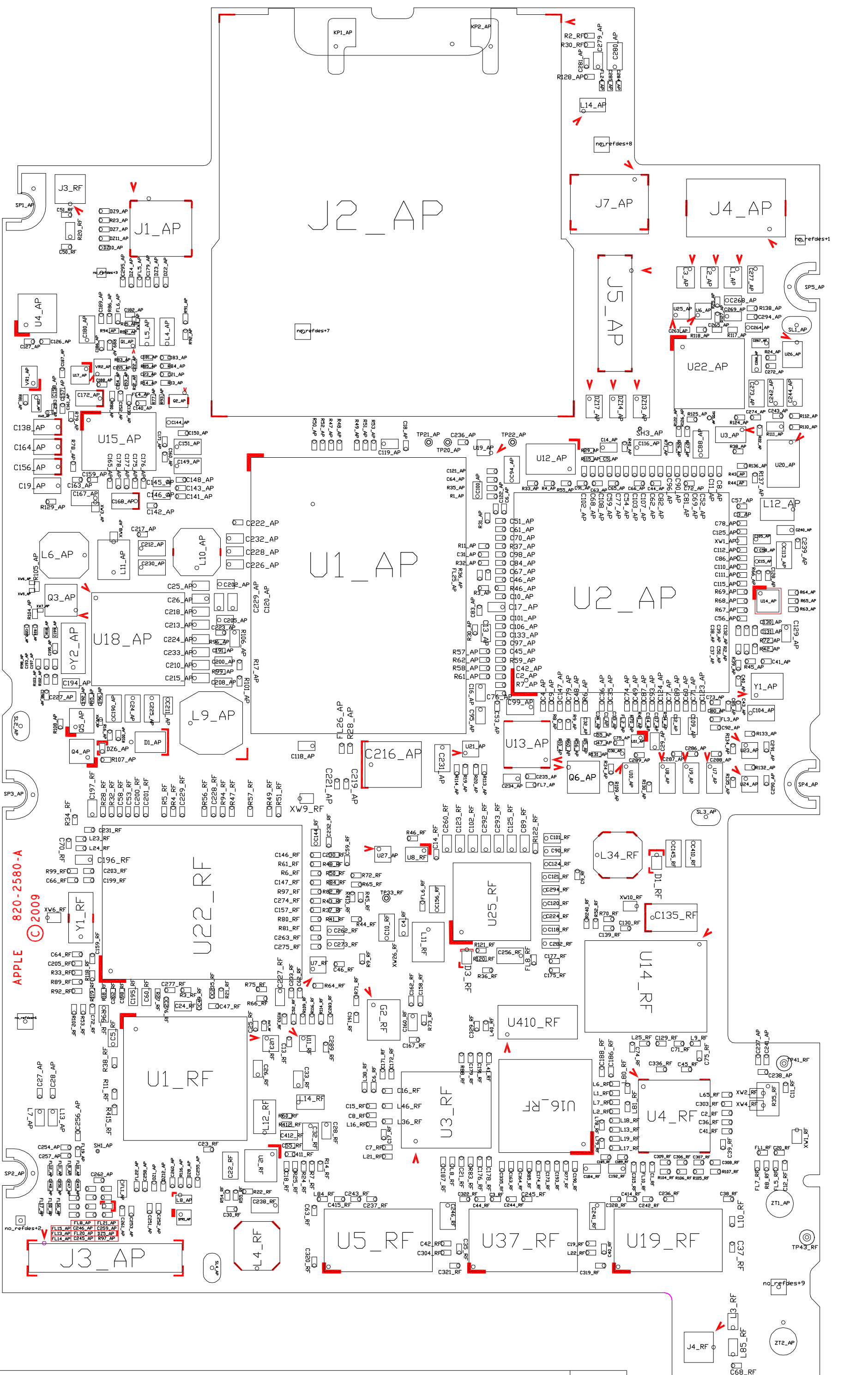
N88 MLB PVT PCBA 零件位置圖 (820-2580-A) Top side
